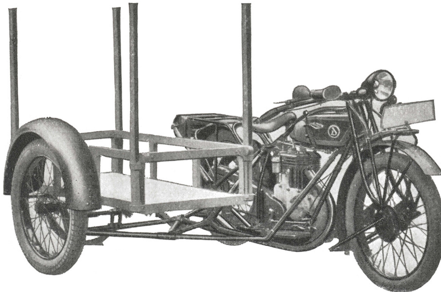
D-Rad Tourenmodell R0/4 mit Pritschen-Beiwagen
