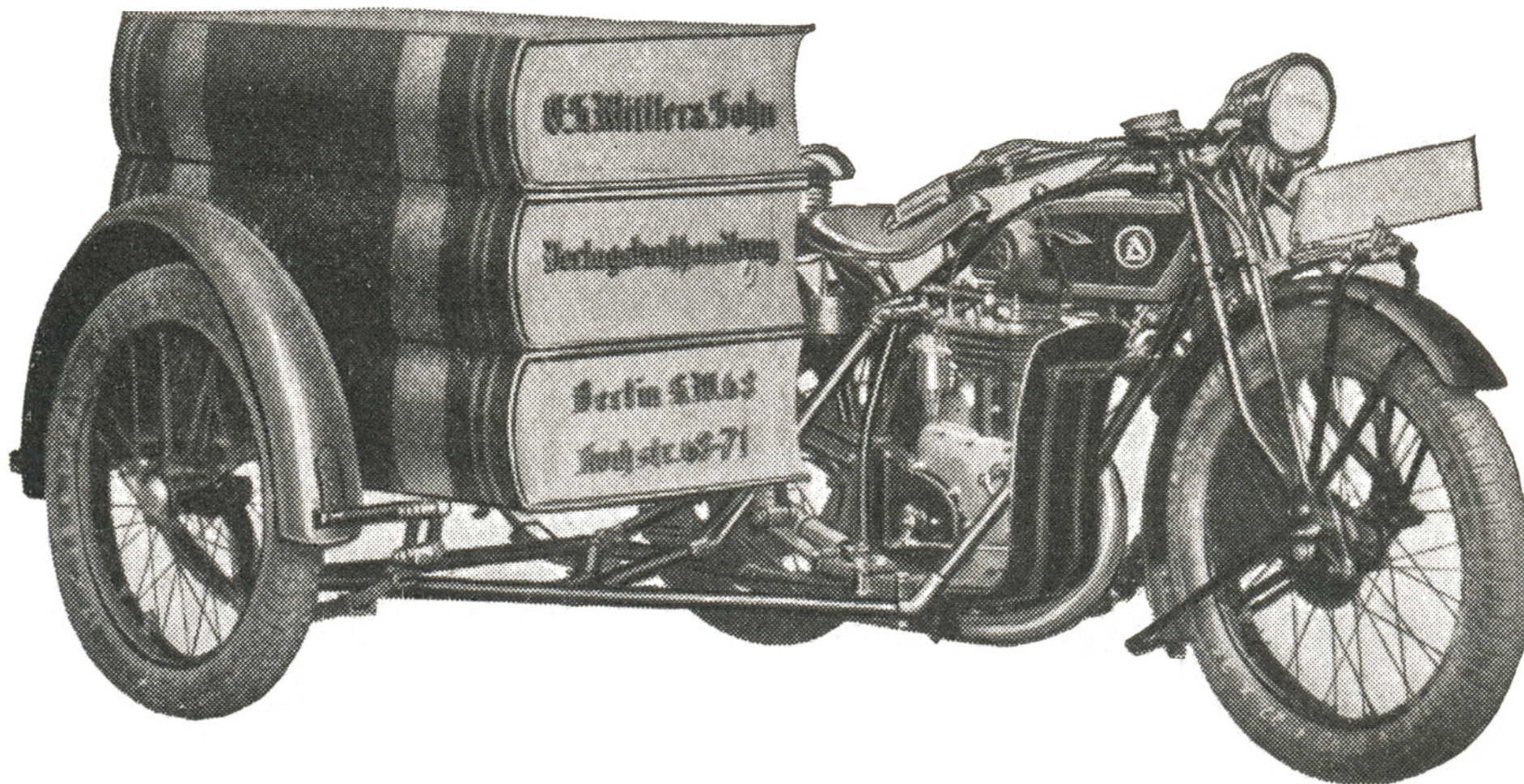
D-Rad Tourenmodell R0/4 mit Beiwagen-Spezialausführung
