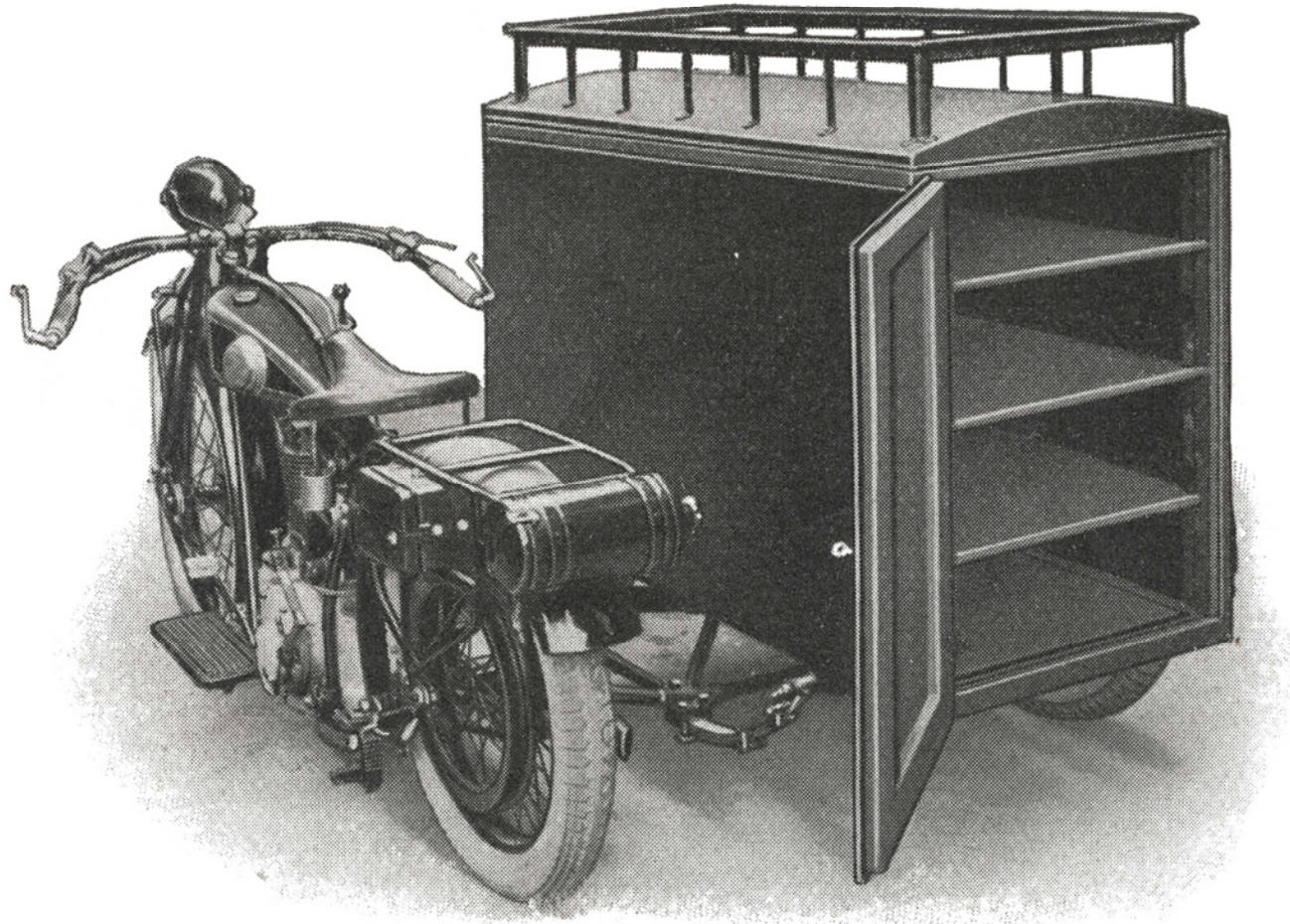
D-Rad mit Lieferbeiwagen, hohe Bauart mit Einlageböden
