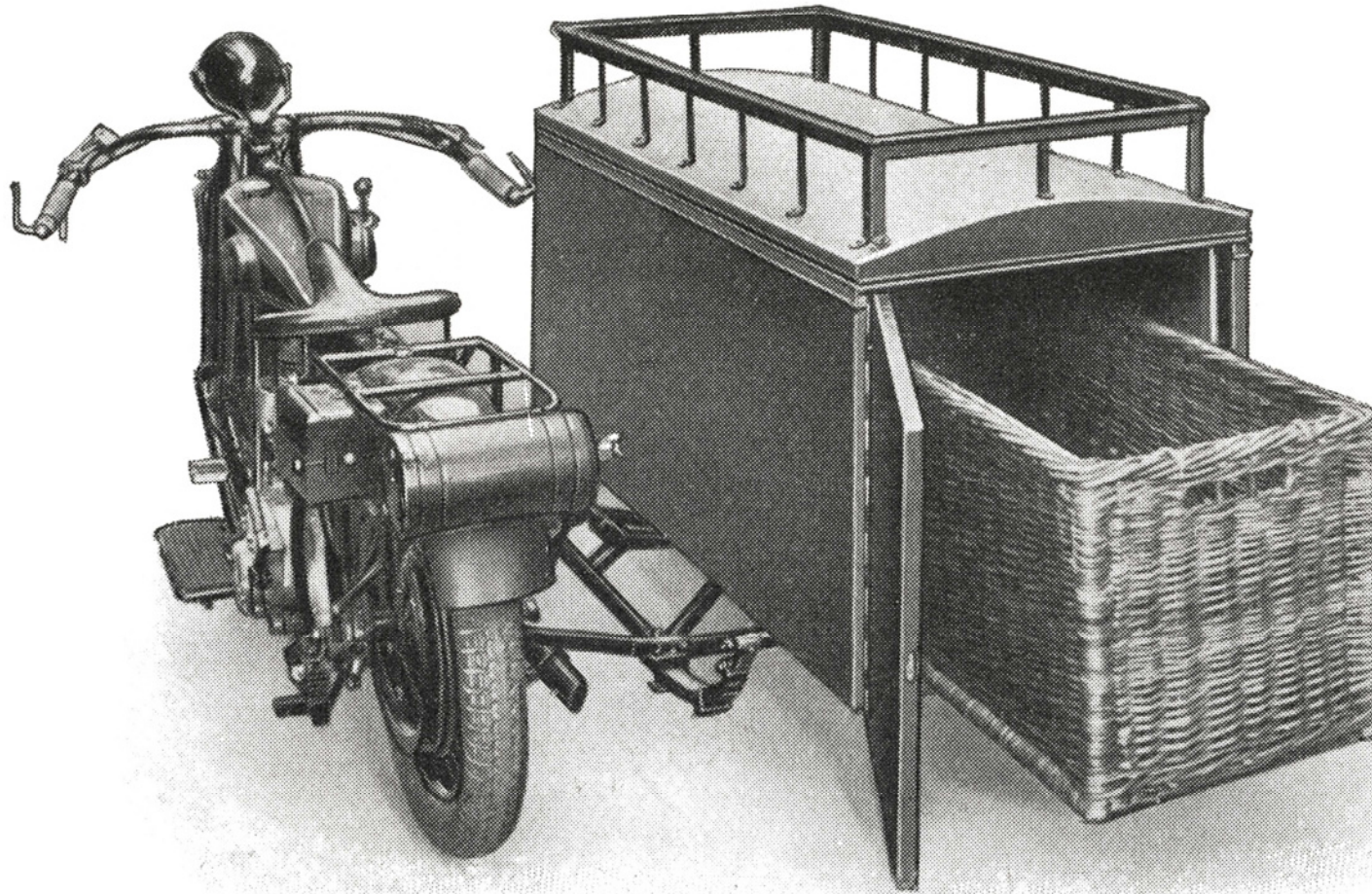
D-Rad Tourenmodell R0/4 mit Lieferbeiwagen, hohe Bauart mit Korb
